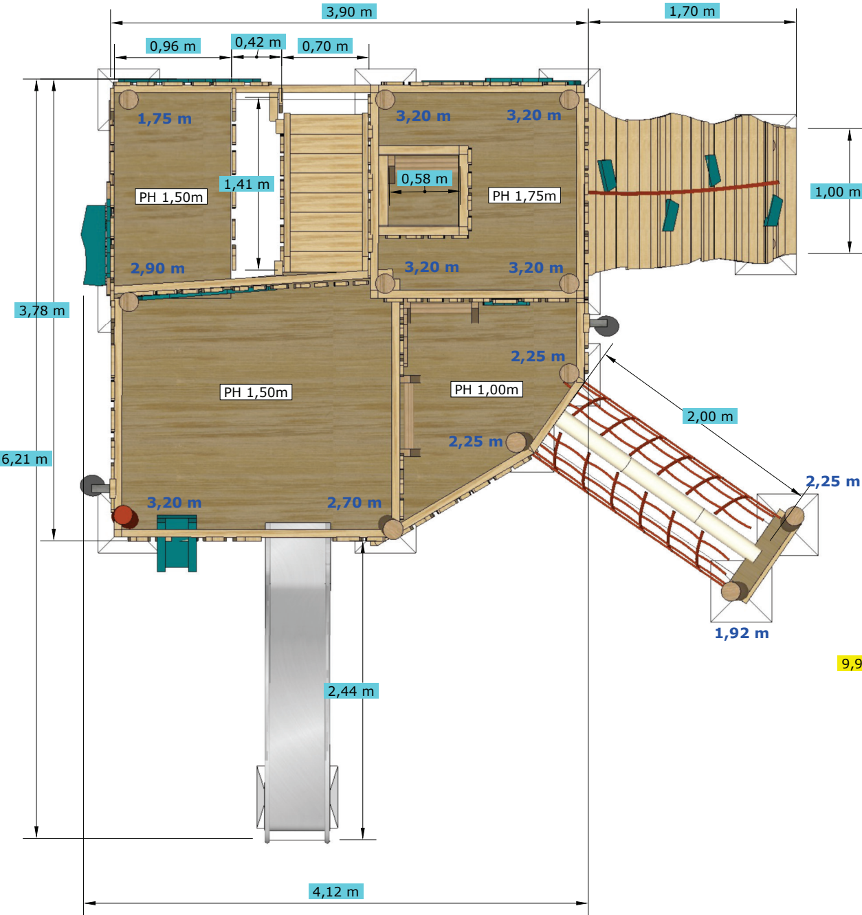
Sicherheitsbereich – Maßstab 1:70
