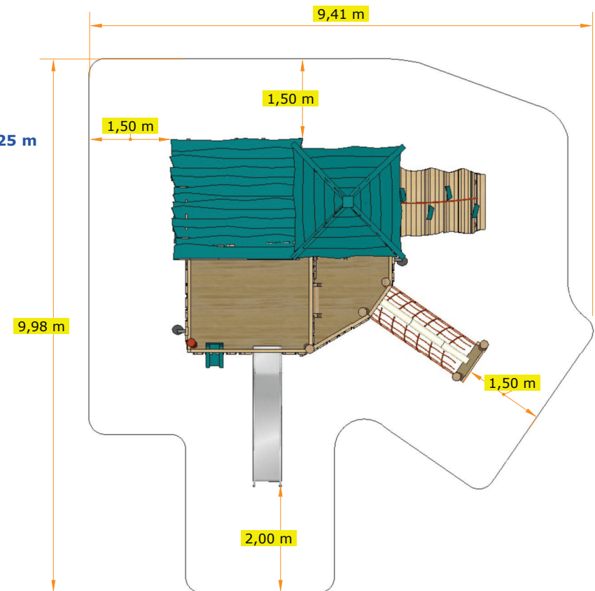
Sicherheitsbereich – Maßstab 1:70
